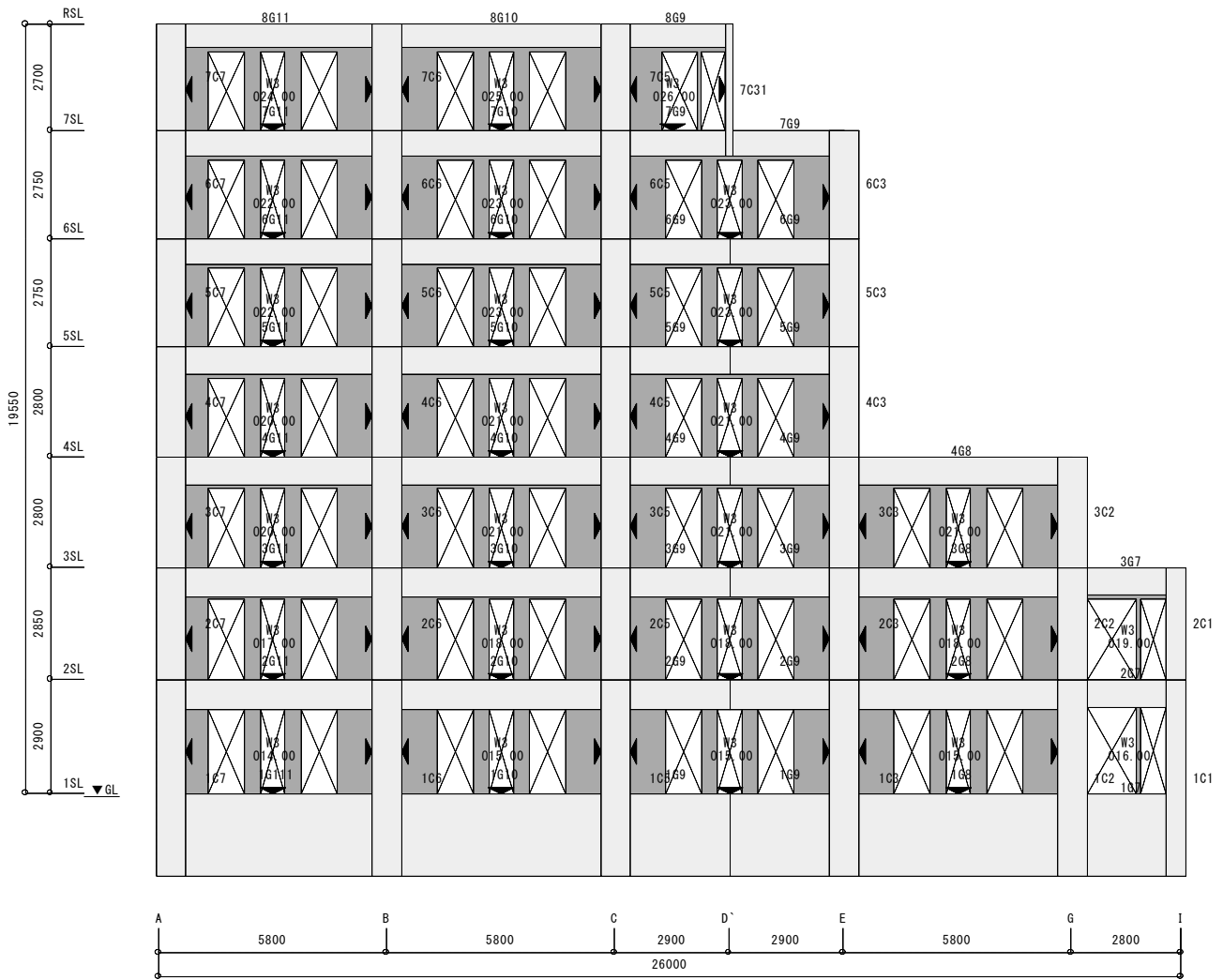
【27フレーム】 スケール : 1/180
