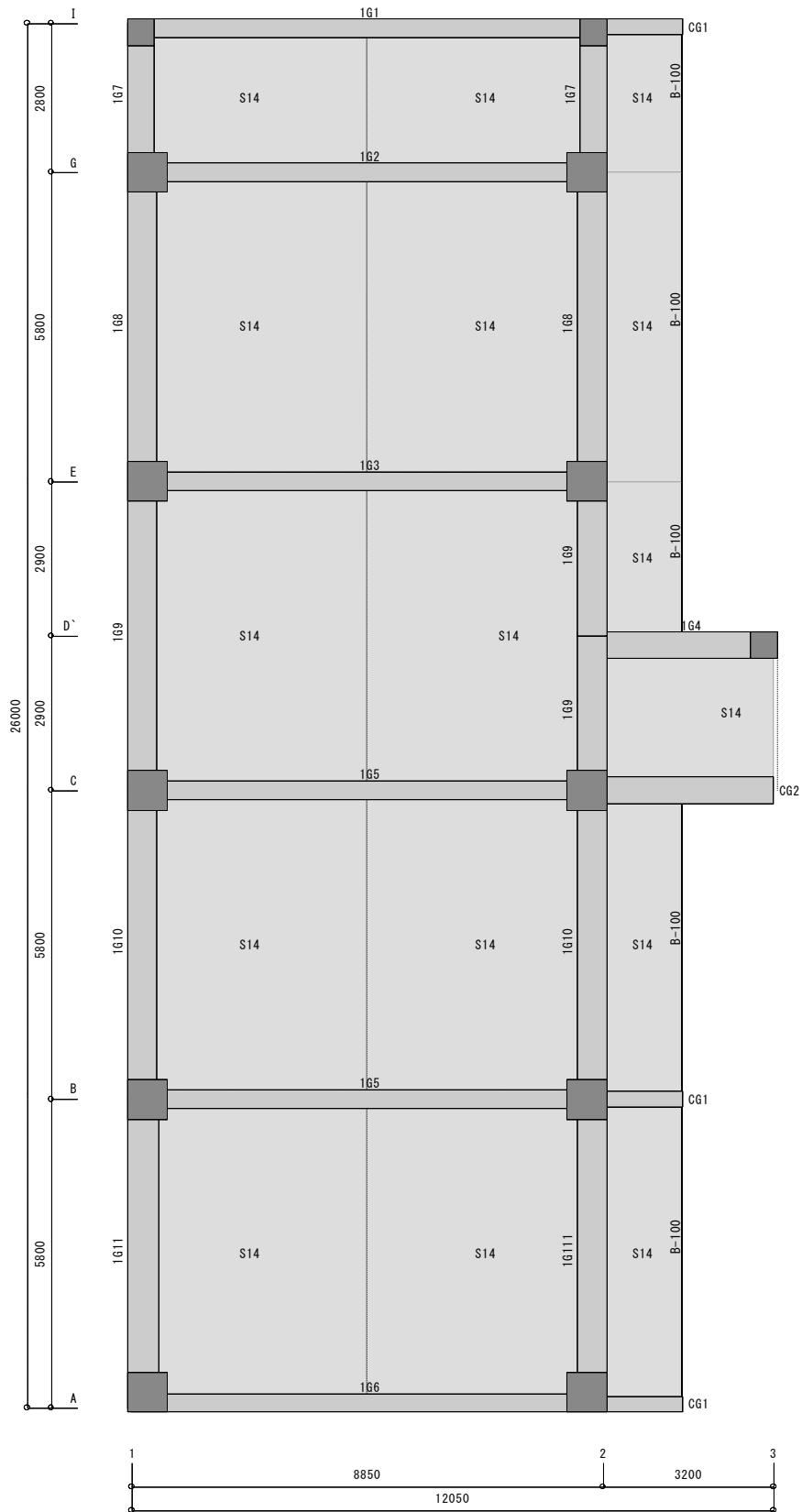
【基礎層】スケール：1/130
