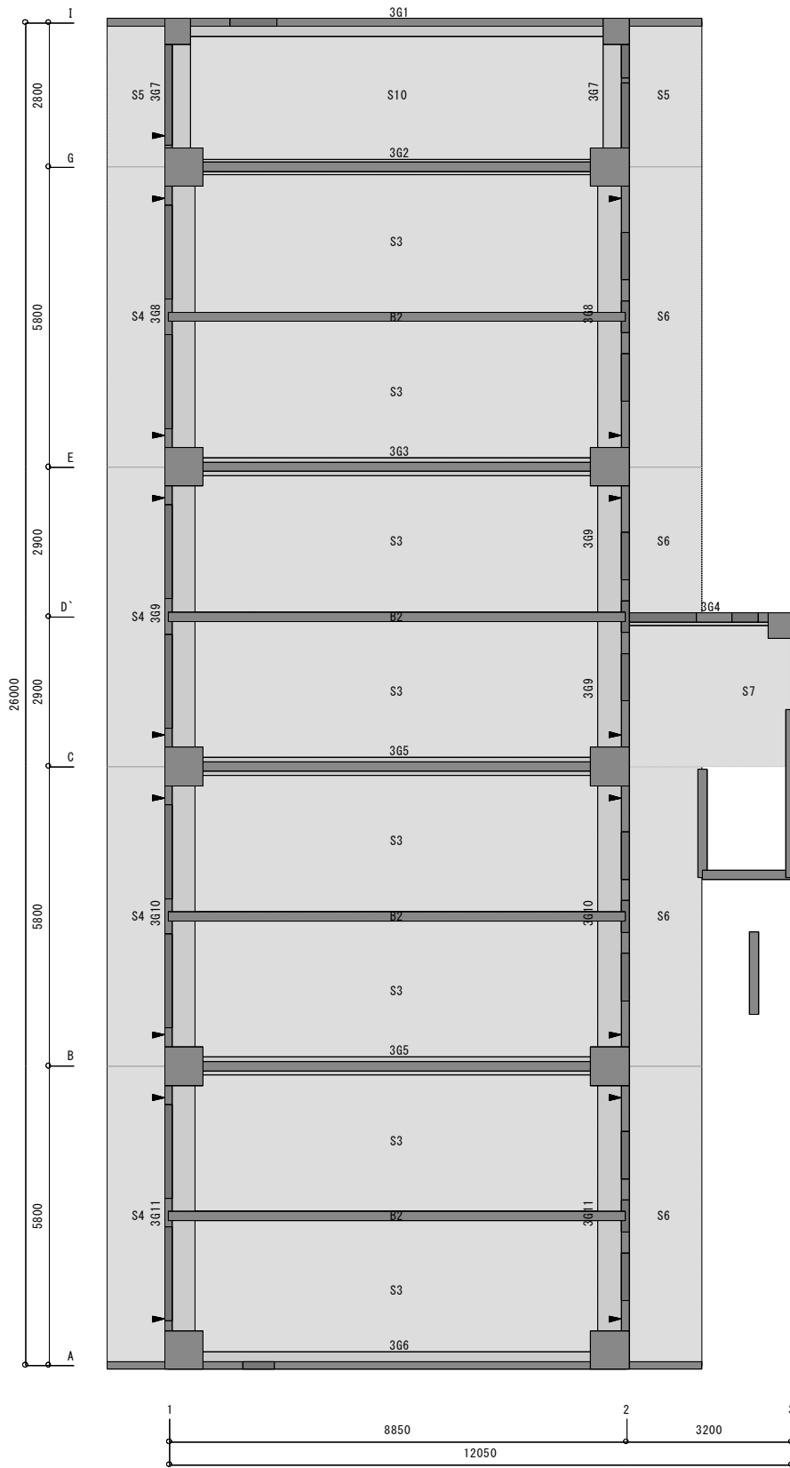
【3SL層 2SL階】スケール：1/130
