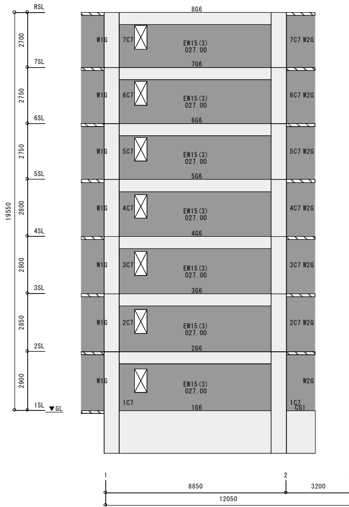
【Aフレーム】 スケール : 1/180
