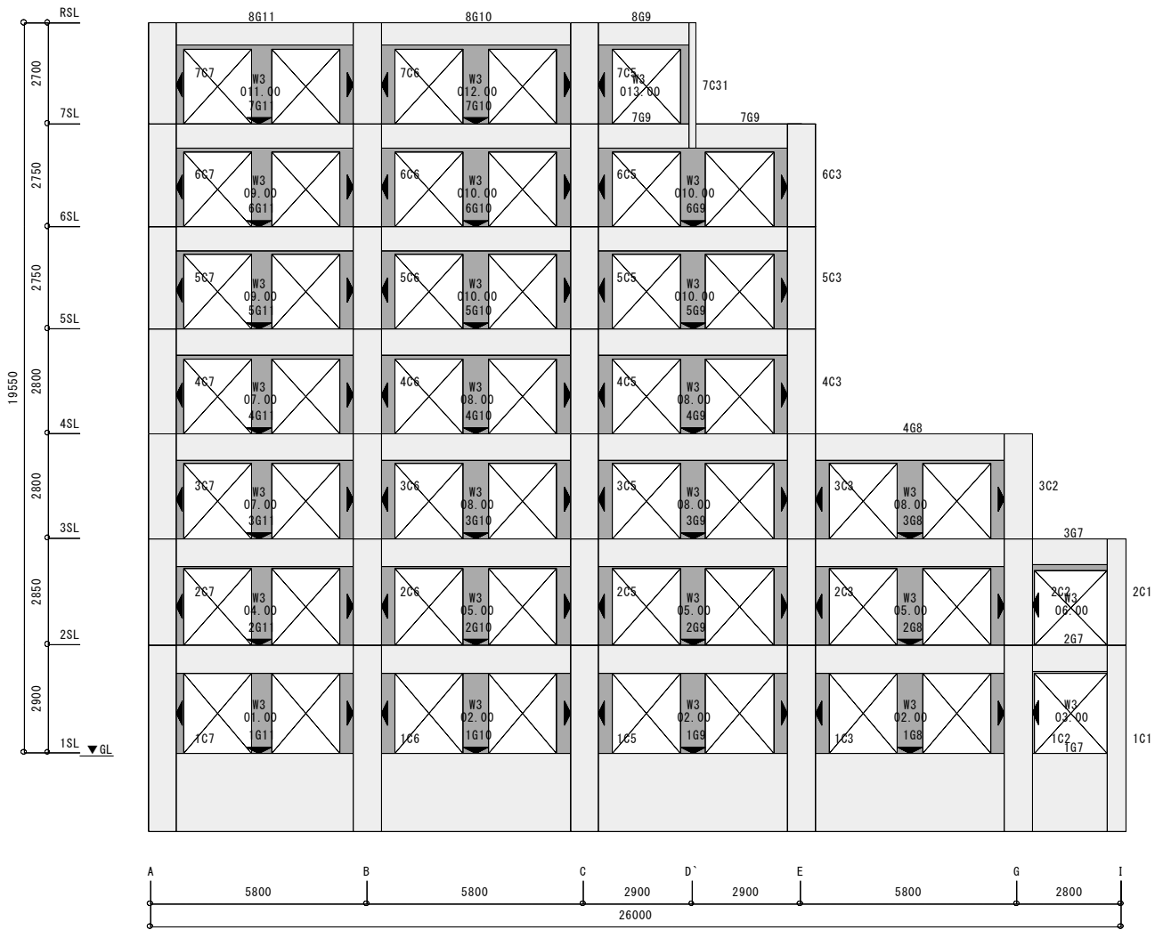
【17レーム】 スケール : 1/180
