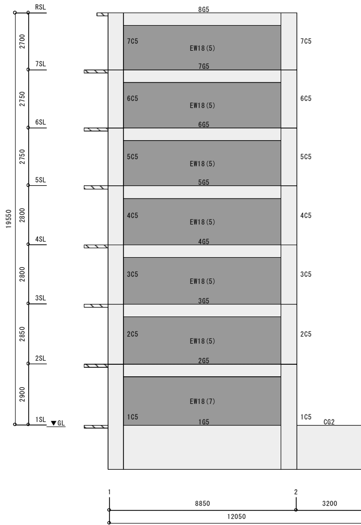
【Cフレーム】 スケール : 1/180
