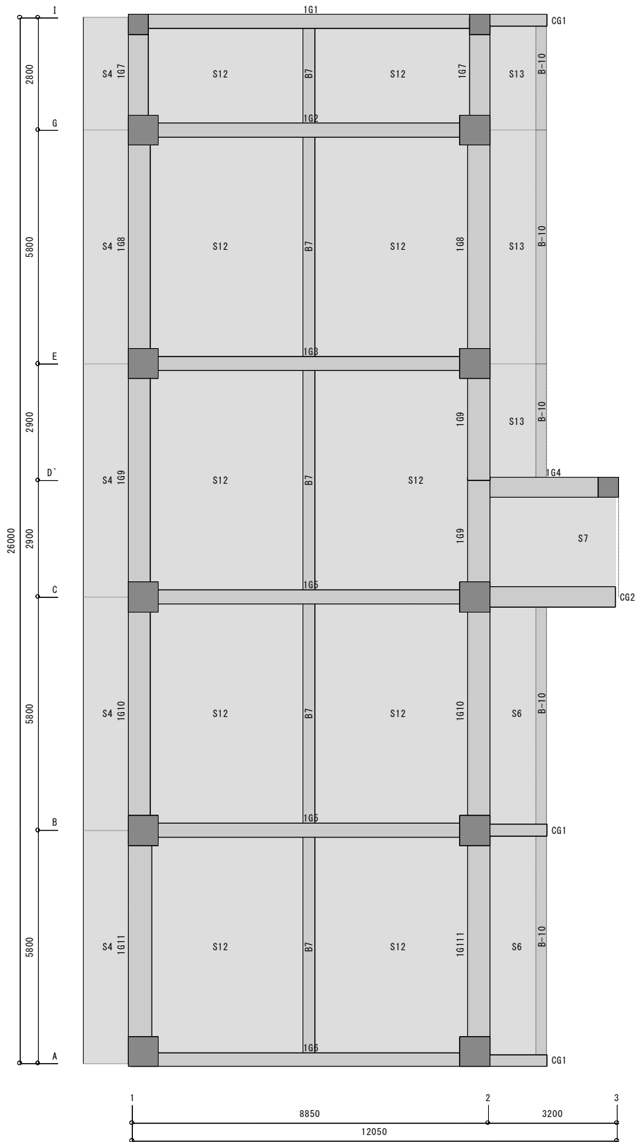
【1SL層 1SL階】スケール：1/130
