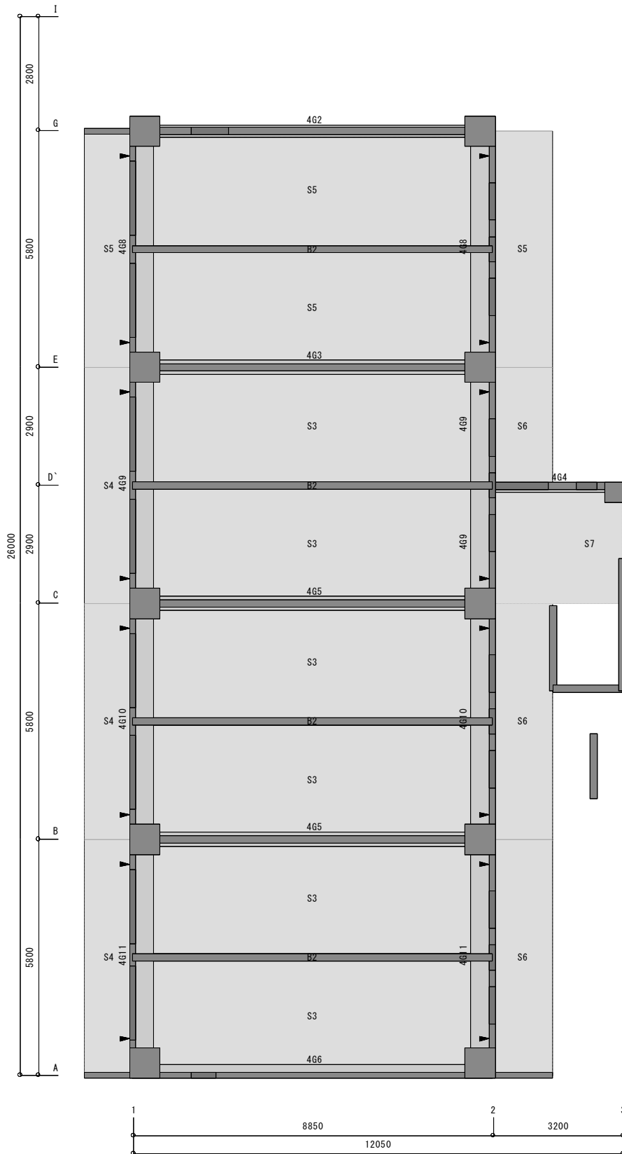
【4SL層 3SL階】スケール：1/130
